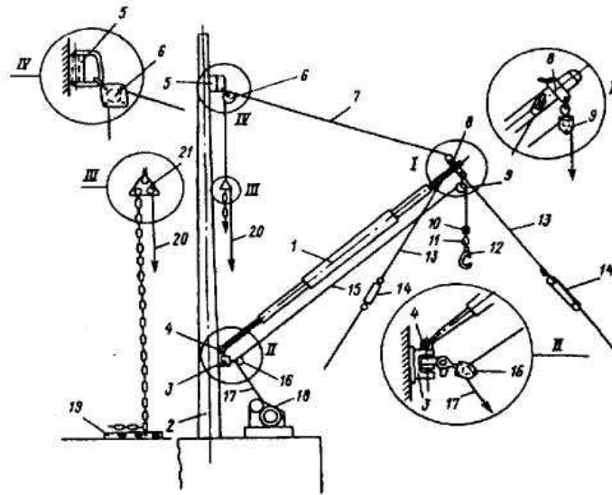
Рис. 5.18. Грузовая стрела:
