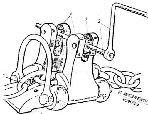
Рис. 9-7. Палубные стопоры.
